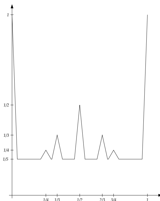
Abbildung 8.2: Die Funktion f_5 aus Beispiel 8.3. Man sieht die „hohen Gipfel“ der Funktion f , allerdings mit der Breite n^{-2} , die im Laufe des Prozesses immer mehr abnehmen wird. Alle anderen Gipfel sind durch den Minimalwert \frac{1}{5} „überflutet“, tauchen aber für hinreichend großes n irgendwann auf.
