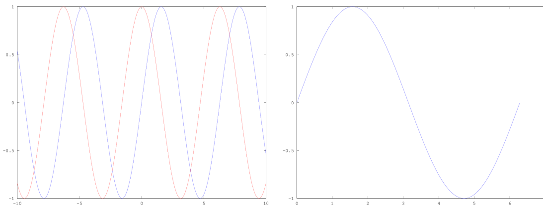
Abbildung 5.1: Links: Cosinus (rot) und Sinus (blau) auf dem Intervall [-10, 10] , so daß man ein paar Schwingungen und die Periodizität sieht. Rechts: Der Sinus auf dem Intervall [0, 2\pi] .
