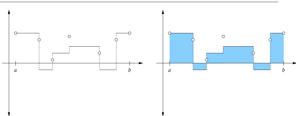
Abbildung 7.1: Eine Treppenfunktion ( links ) mit den Funktionswerten an den Unterteilungsstellen und deren Integral in geometrischer Interpretation ( rechts ): Man nimmt einfach die vorzeichenbehafteten Flächen der von der Funktion und der x -Achse gebildeten Rechtecke und summiert diese auf. Dabei spielen die „Kringel“ keine Rolle mehr.
