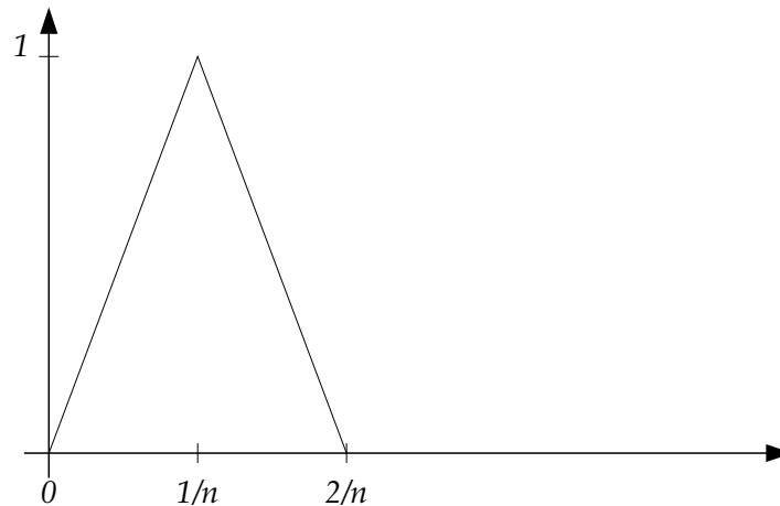
Abbildung 8.1: Einfachstes Beispiel einer punktweise, aber nicht gleichmäßig konvergenten Funktionenfolge. Das „Dach“ rückt für n \rightarrow \infty immer weiter nach links.
