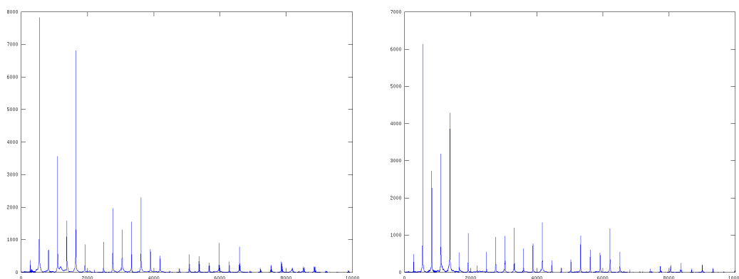
Abbildung 8.4: Klangfarben zweier verschiedener Pianos. Diese Werte sind aber mit Vorsicht zu sehen, denn der Ton eines Pianos ist eben nicht periodisch sondern klingt exponentiell ab.
